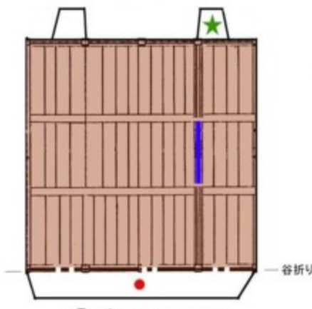
⑰勝手門天井
